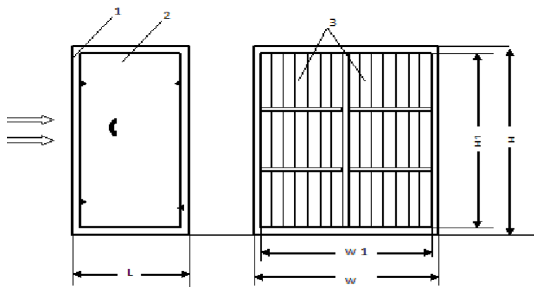
Рис.1 Схема МФФ 1-корпус; 2 – сервисная панель; 3 – панельные фильтры
